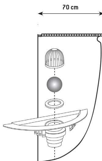
Montaż blokady zapachów MEASTOP w doświetlaczach MEAMULTINORM, głębokość (odstęp od muru) 70 cm
